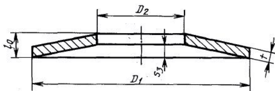
Пружина типа 3
