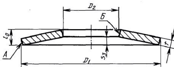
Пружина типа 1
