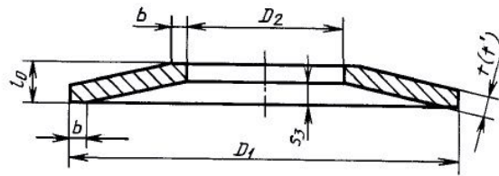
Пружина типа 4
