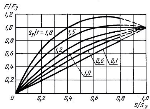
Зависимость характеристики «сила-деформация» от отношения \frac{s_3}{t}
