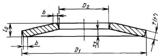
Пружина типа 2
